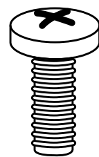
M8x30 (قطع 4)
